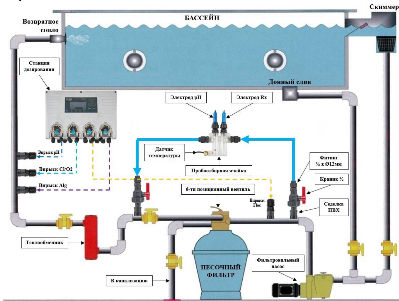
Гидравлическая схема подключения №1
