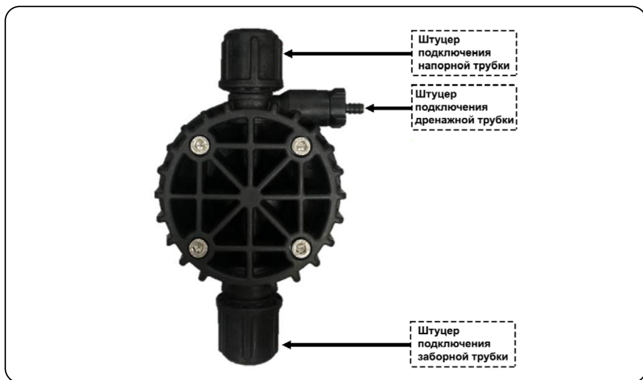
Рис.4 - Схема подключения трубок к мембранному насосу
