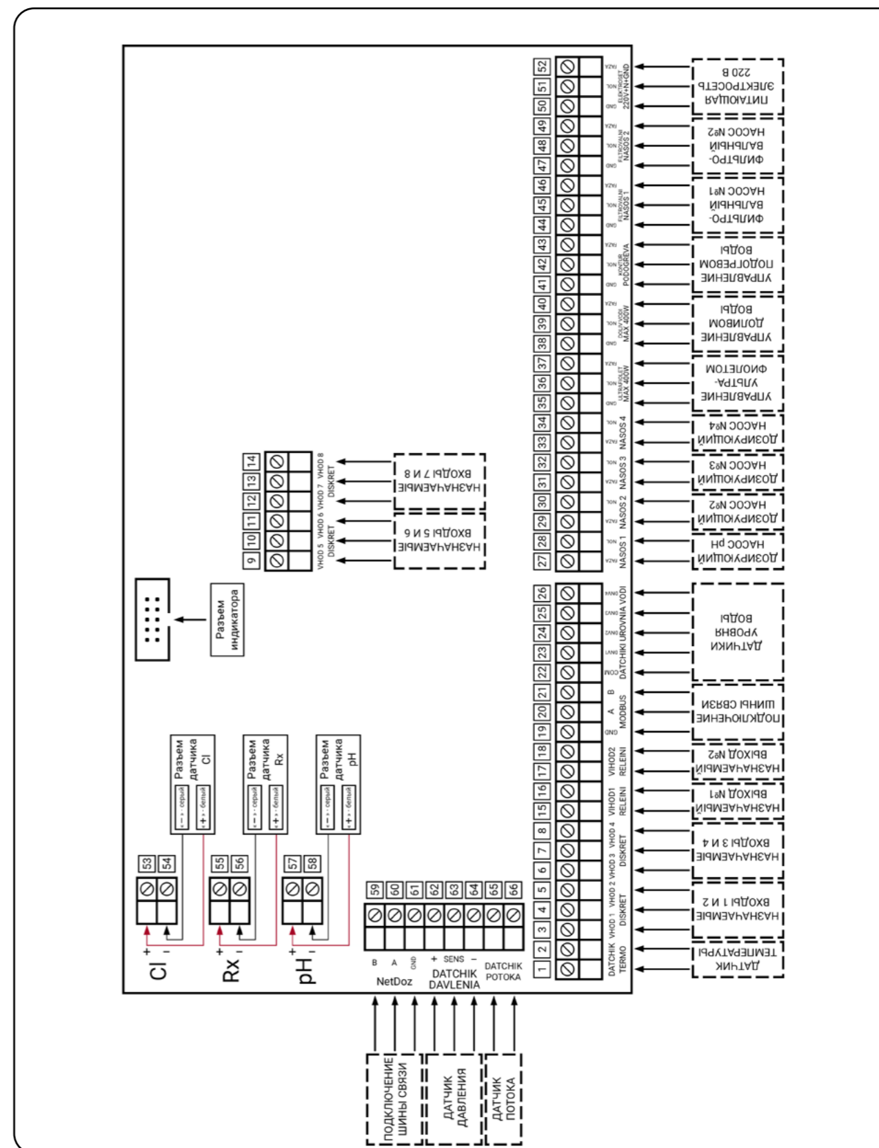
Рис.5 - Электрические подключения DOMINATOR-M PRO
