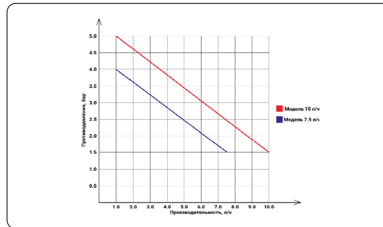
Рис.3 - График производительности мембранных насосов
