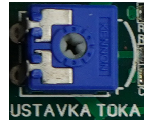
Рисунок 3 - Подстроечное сопротивление
