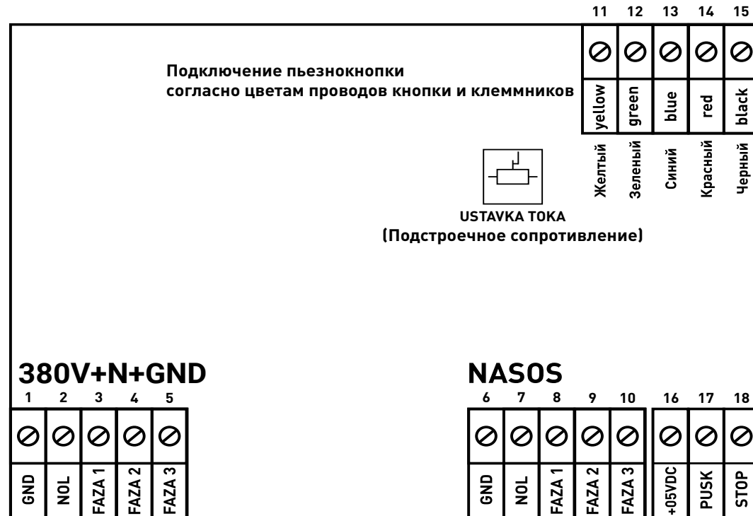
Рисунок 2 - Схема клеммников платы
